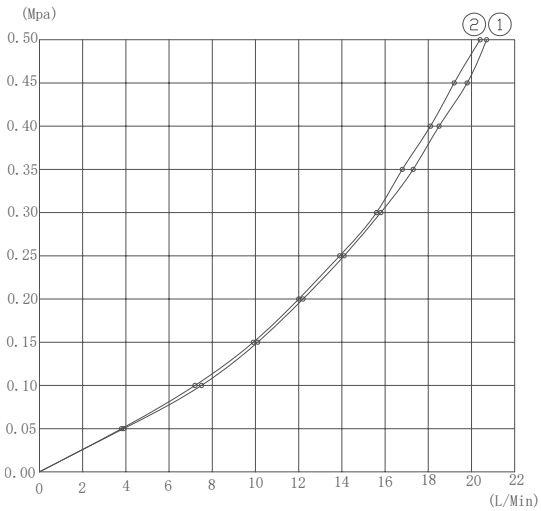
流量曲线图 ①顶喷出水 ②手持出水
