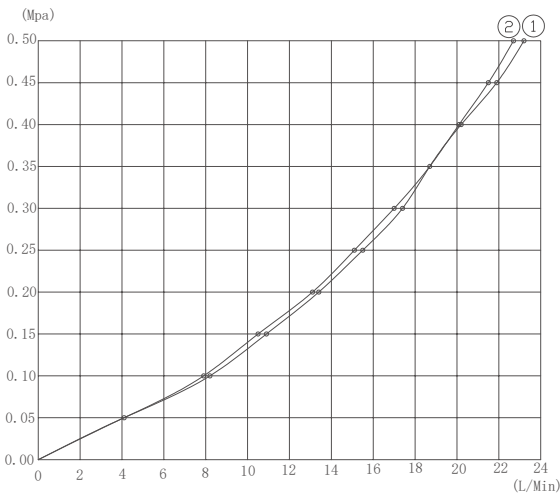
流量曲线图
