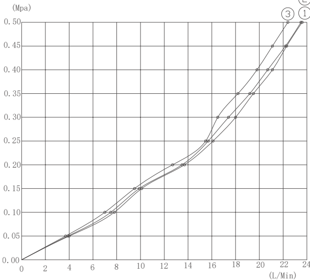
流量曲线图
