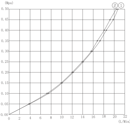
流量曲线图
