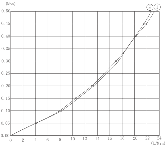
流量曲线图 ①顶喷出水 ②手持出水
