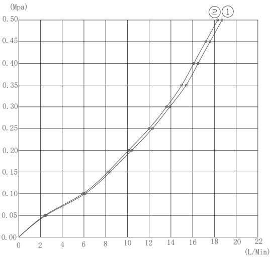
流量曲线图
