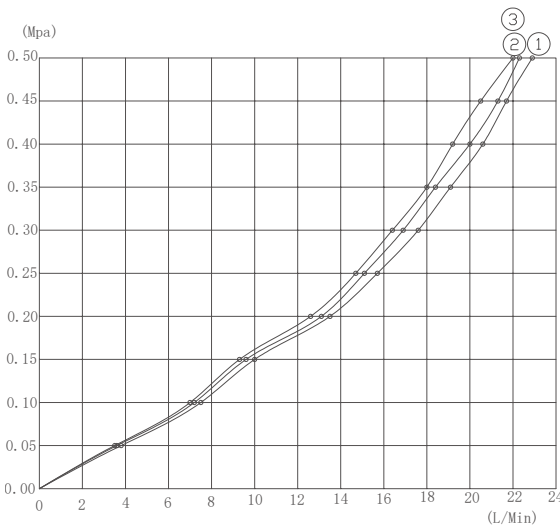
流量曲线图 ①手持出水 ②顶喷雨淋水 ③顶喷瀑布水
