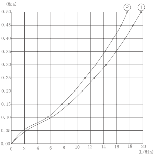
流量曲线图 ①顶喷出水 ②手持出水
